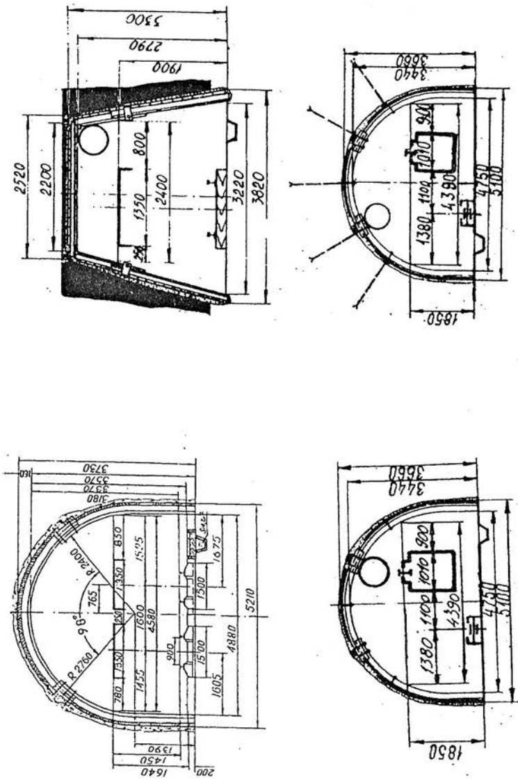
Рис. П. 3.2. Сечение кварцлага (а), вентиляционного штрэка (б) и бремсберга (в, г)
